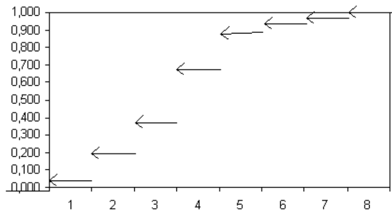
Рис. 6.2. График эмпирической функции распределения
