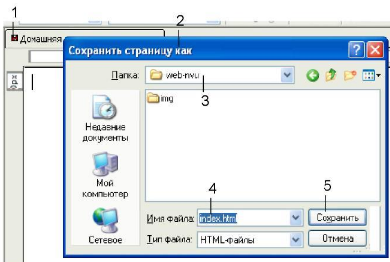
Рисунок 4.2 – Сохранение web-страницы
