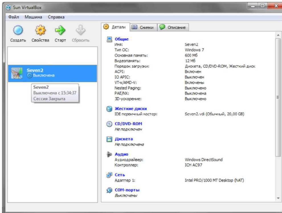
Рис. 7. Главное окно программы VirtualBox.
