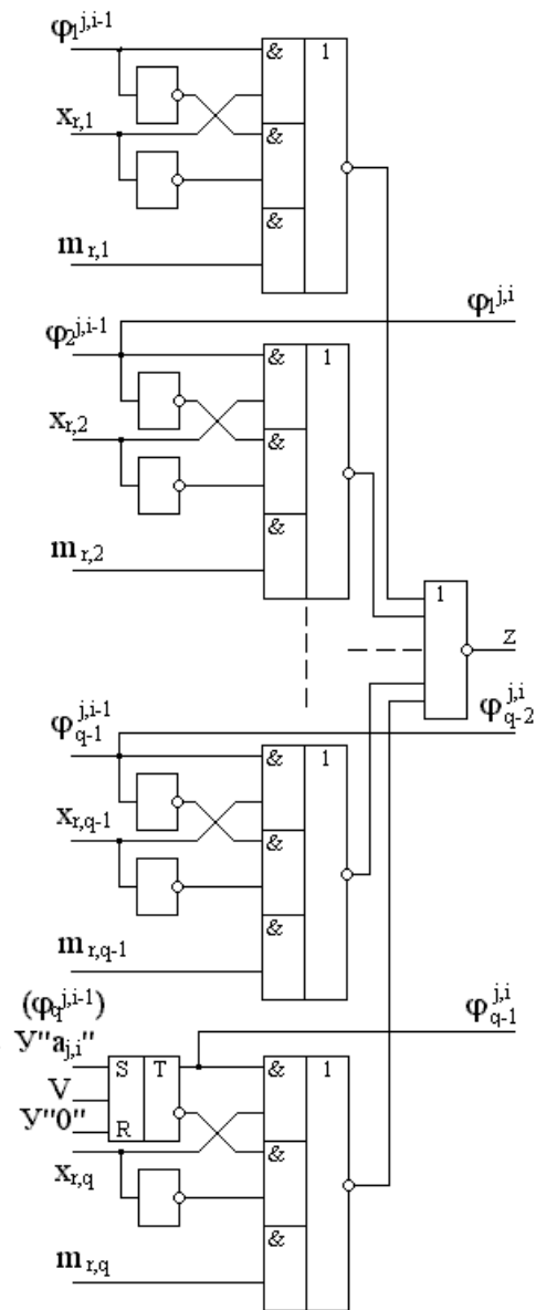
Рис. 1.35. Базовый ассоциативный модуль двумерного поиска
