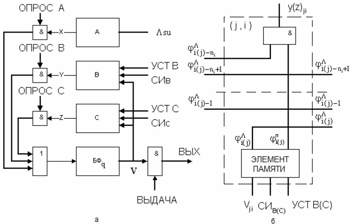
Рис. 1.43. Организация обрабатывающей части мчп процессора (а) и элемента среды (б)
