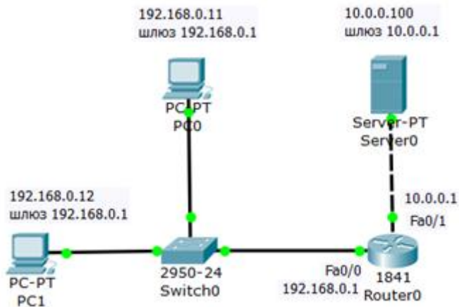
Рис. 9.1. Схема сети
