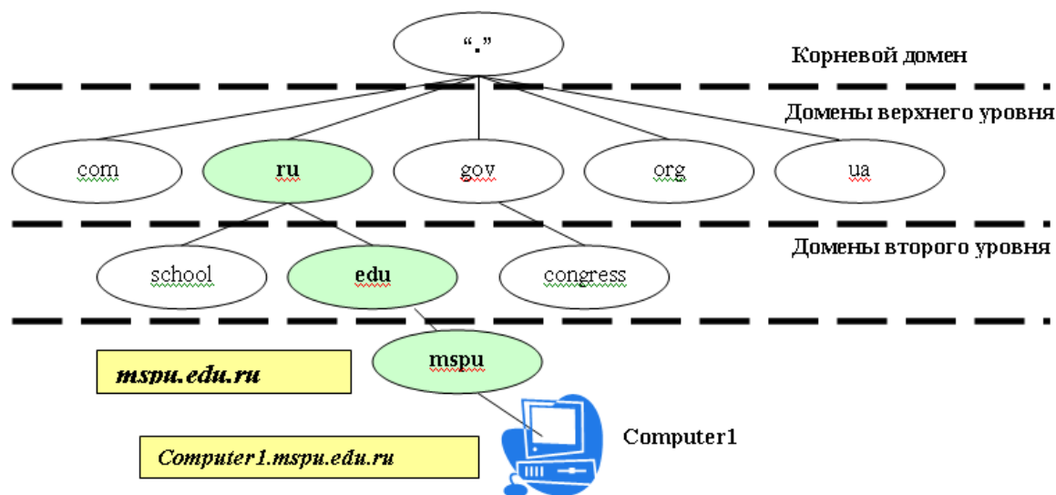
Рис. 2. Пример образования иерархии пространства имен домена
