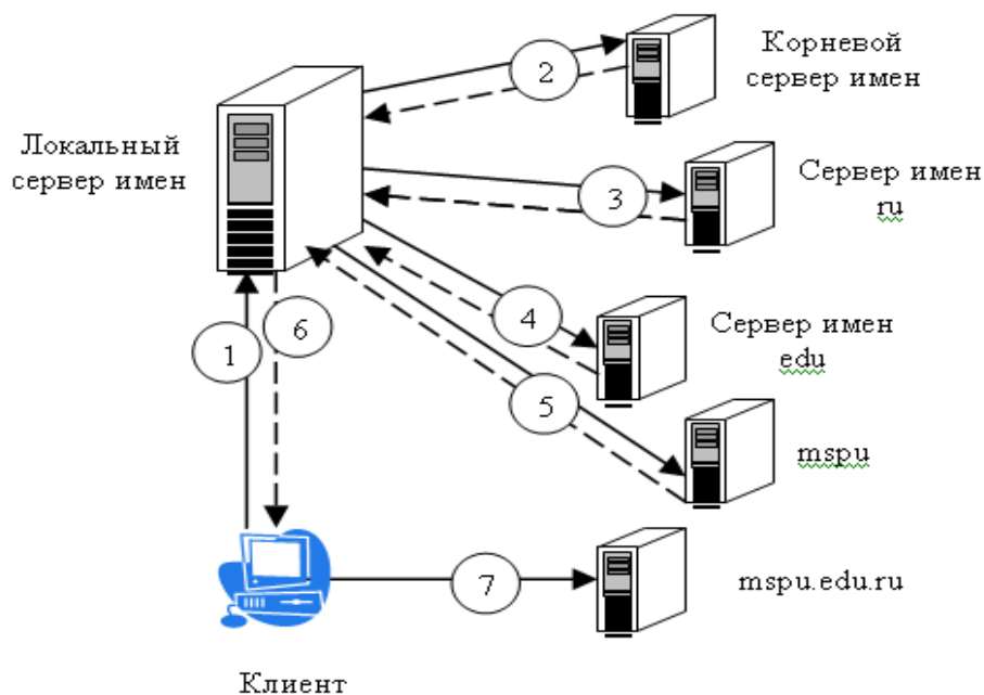
Рис. 3. Процесс разрешения адреса
