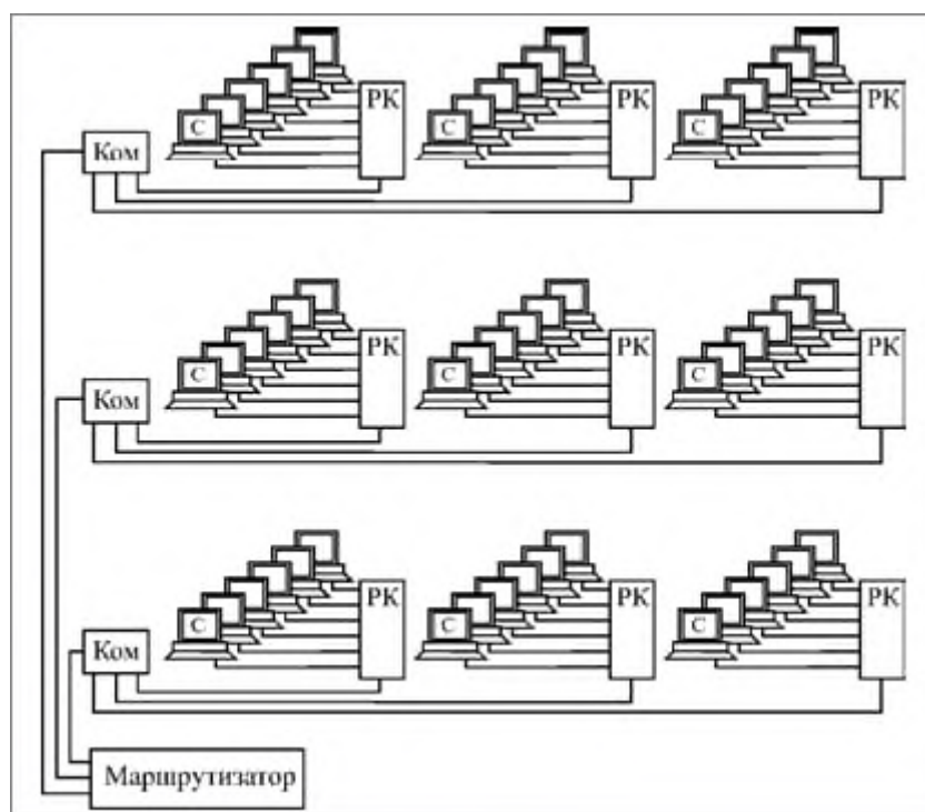
Рис. 1. Структура сети предприятия (С – серверы рабочих групп, ПК – репитерные концентраторы, Ком – коммутаторы )
