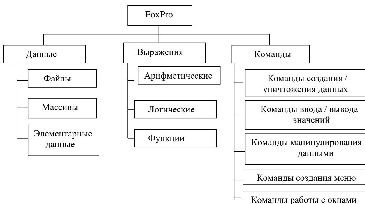
Рис.7.1. Архитектура FoxPro
