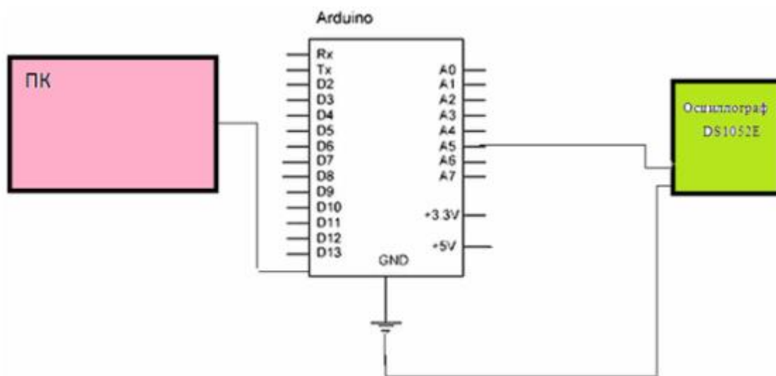
Рисунок 1 – Структурная схема подключения компьютера и осциллографа к микроконтроллеру Arduino Uno
