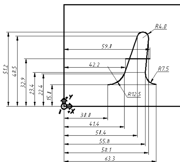
Рисунок 2 – Эскиз детали
