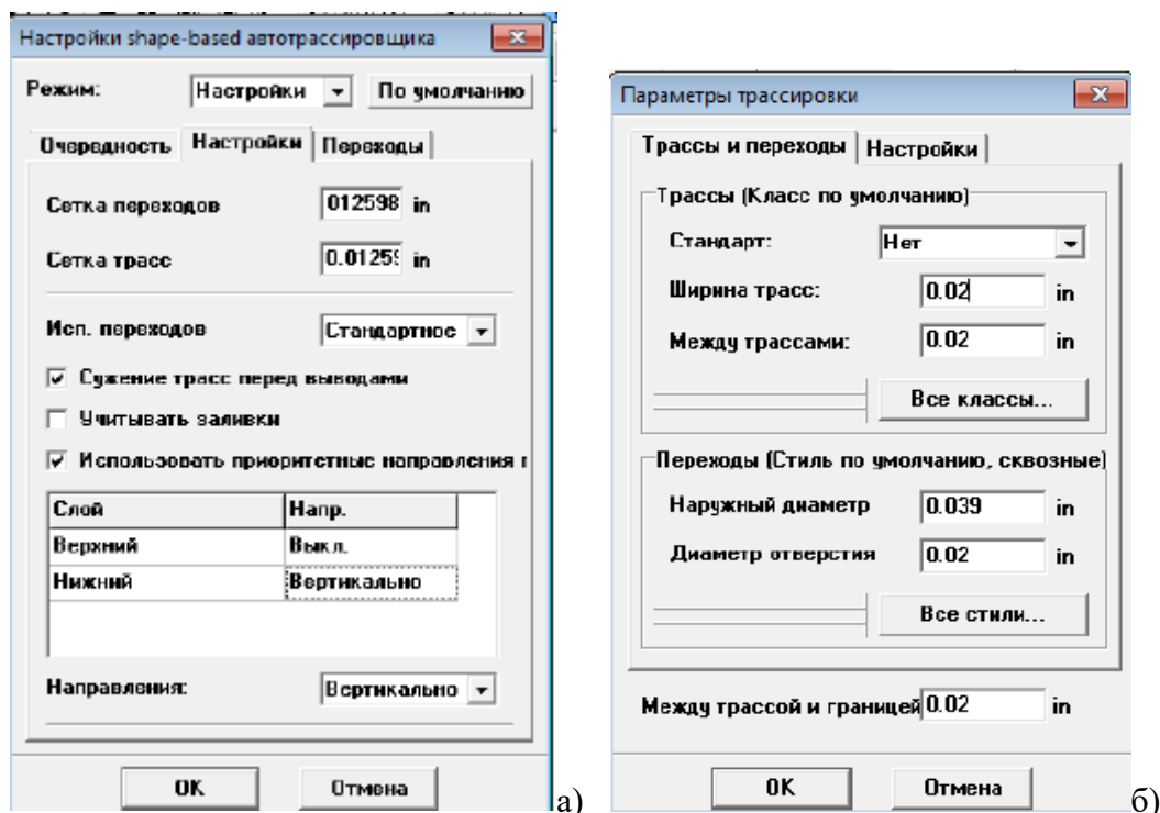
Рисунок 6 – Задание параметров трассировки: а) настройки share-based автотрассировщика; б) настройка параметров трассировки
