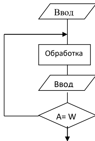
а) цикл с постусловием
