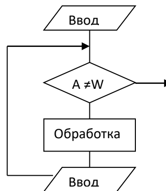
б) цикл с предусловием
